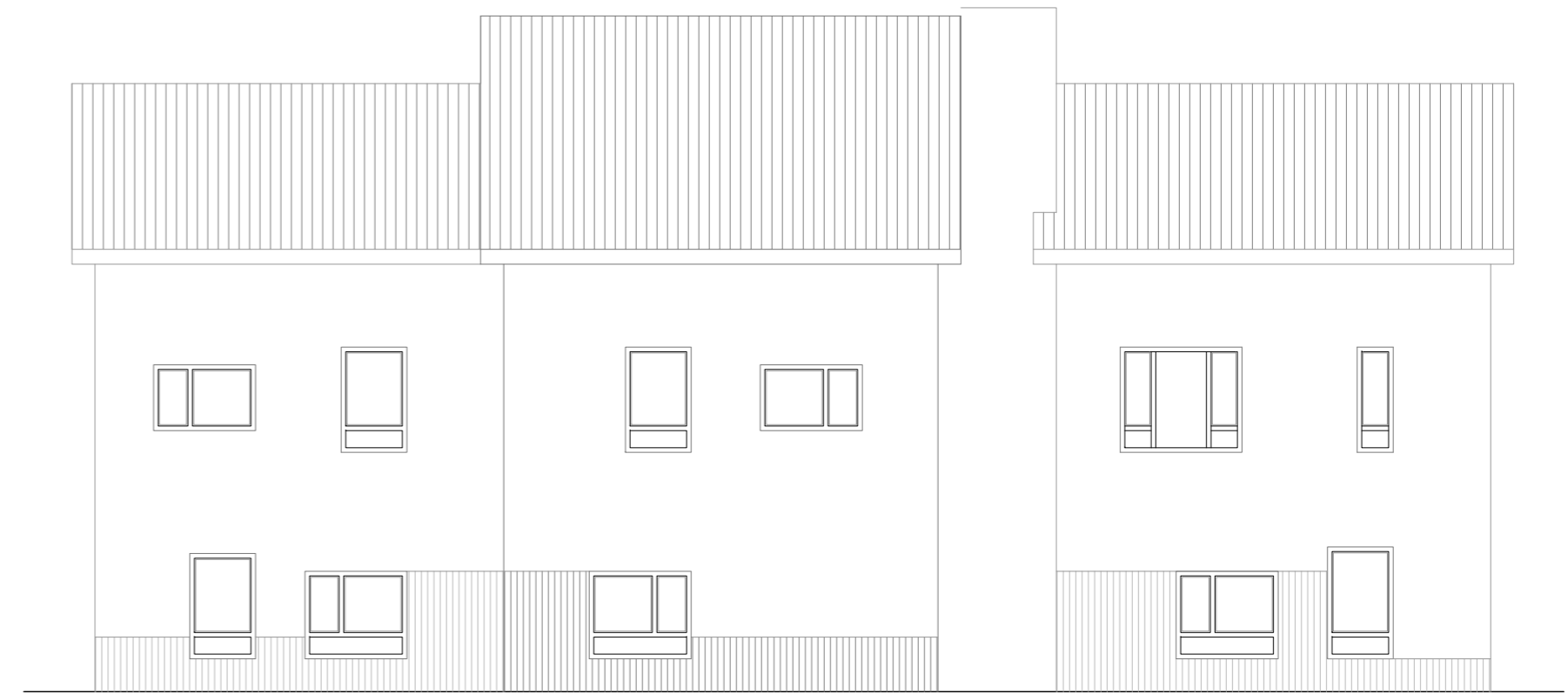
ALZADO NORESTE
