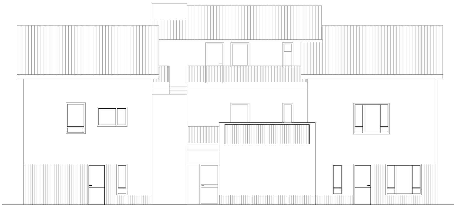
ALZADO SUROESTE
